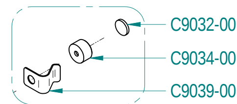
DET. B
