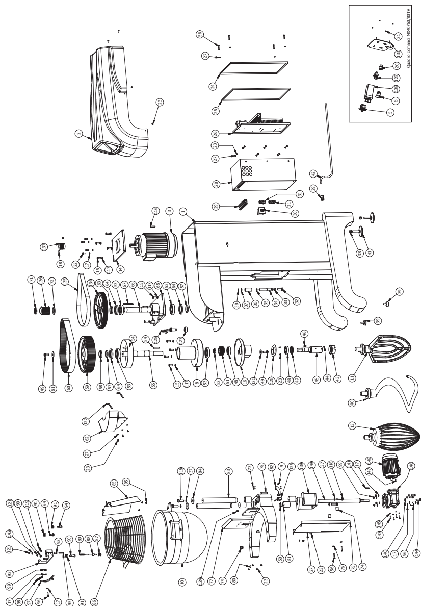
FIG. / РИС. 32 - MX40/60/80 TV Parti di ricambio / Replacement parts / Pieces de rechange / Repuestos / Запасные части
