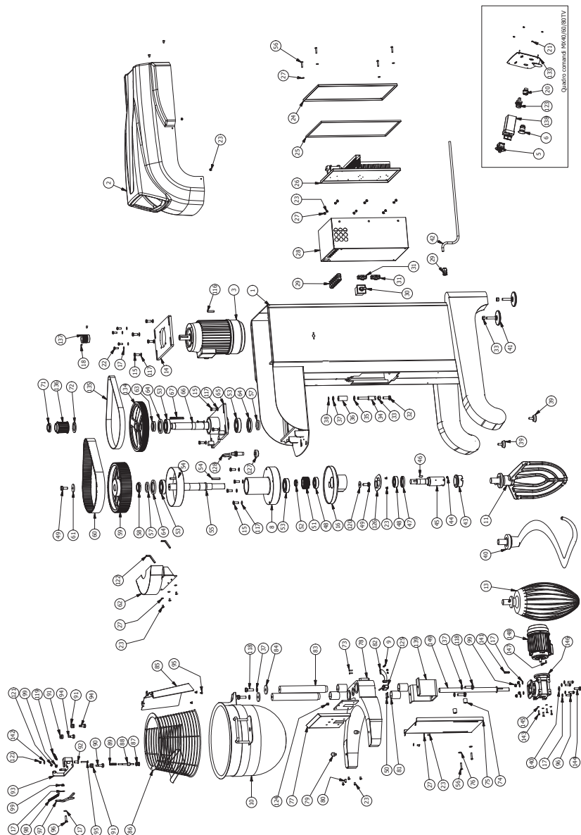
FIG. / PИC. 32 - MX40/60/80 TV Parti di ricambio / Replacement parts / Pieces de rechange / Repuestos / Запасные части
