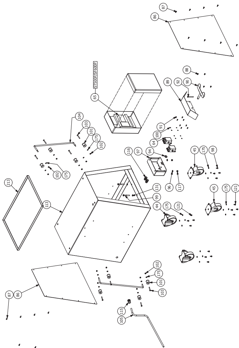
FIG. / ABB. / РИС. 24 - SB500-ST500 Parti di ricambio / Spare parts / Pieces de rechange / Repuestos / Ersatzteile / Запасные части
