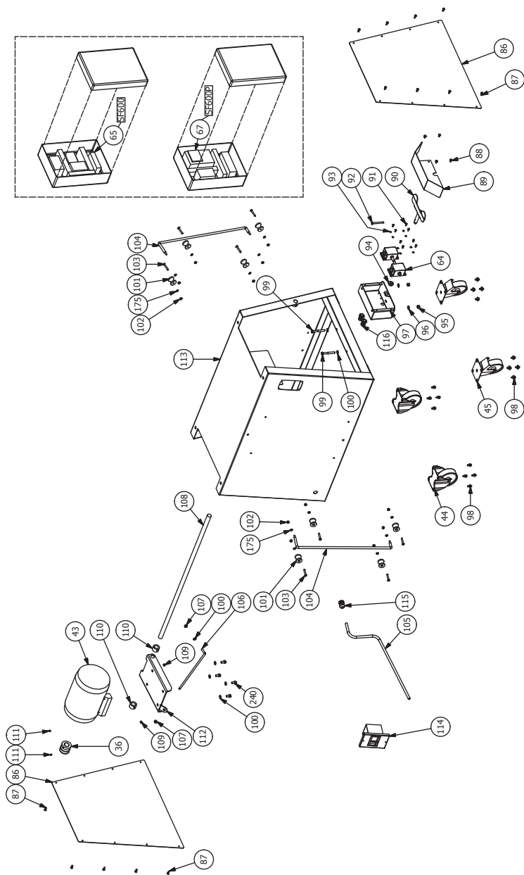
FIG. / ABB. / PИC. 28 - SF500 Parti di ricambio / Spare parts / Pieces de rechange / Repuestos / Ersatzteile / Запасные части
