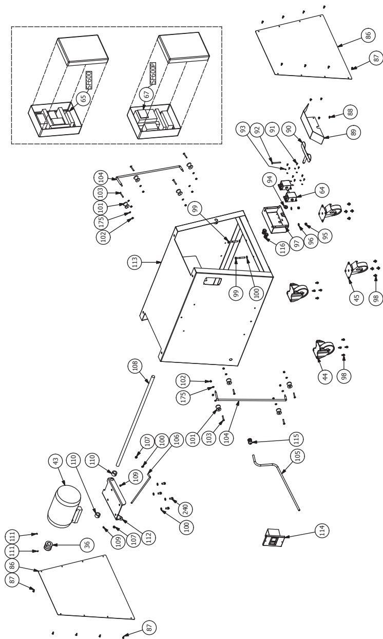
FIG. / ABB. / PИC. 28 - SF5000 Parti di ricambio / Spare parts / Pieces de rechange / Repuestos / Ersatzteile / Запасные части
