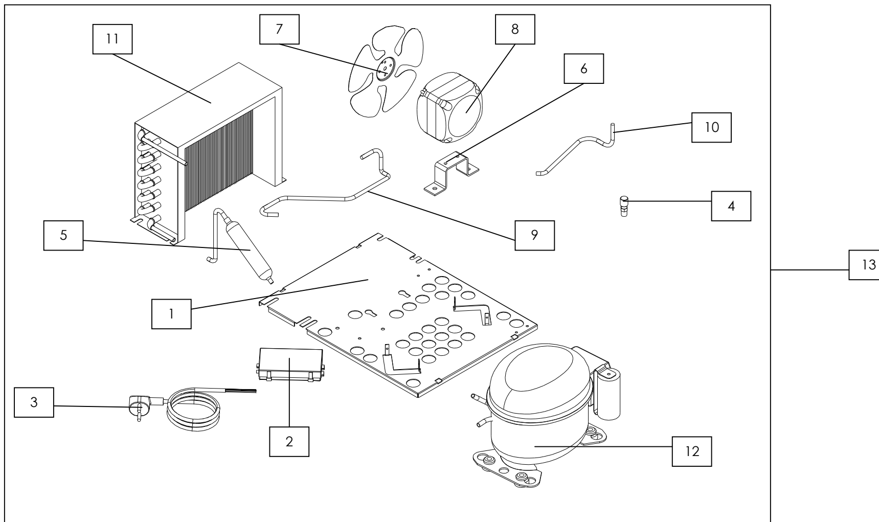
COMPRESSORS GROUPS / GROUPES COMPRESSEURS/ KOMPRESSOREINHEIT
