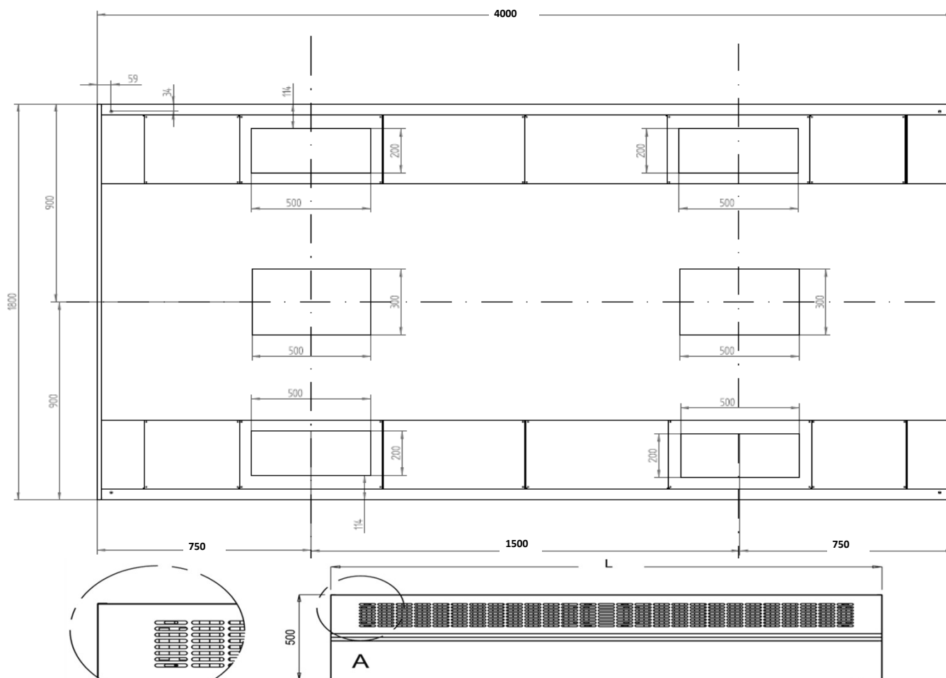
DETTAGLIO A
