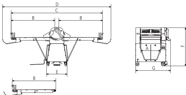
SF600-85/100/120/140
