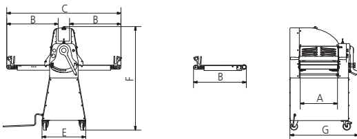
ST500-50/70
