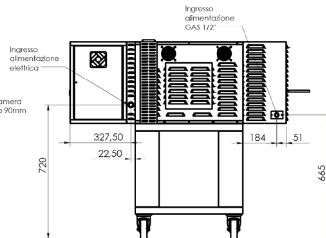
VISTA A SCALA 1 : 20
