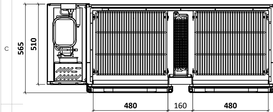
A-A (1 : 14)
