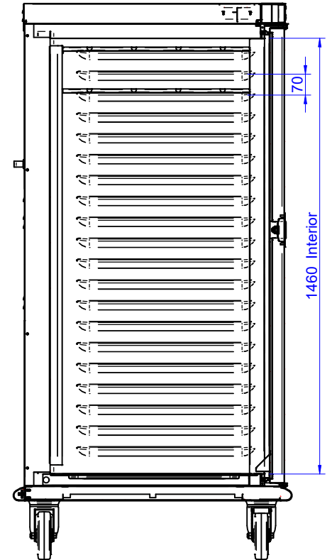
CORTE B-B
