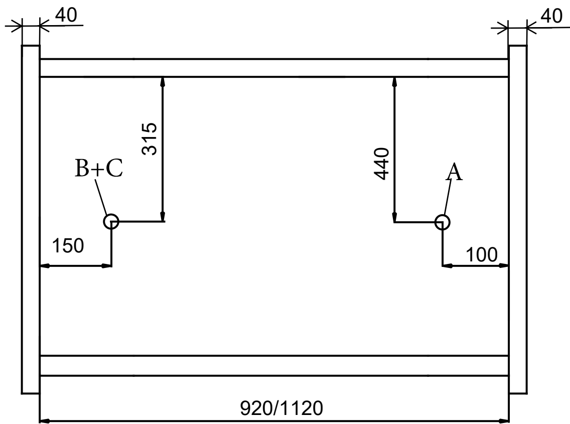
LATO CLIENTE VISTO DALL'ALTO
