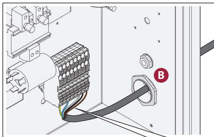
Exemple indicatif d'insertion des câbles de raccordement
