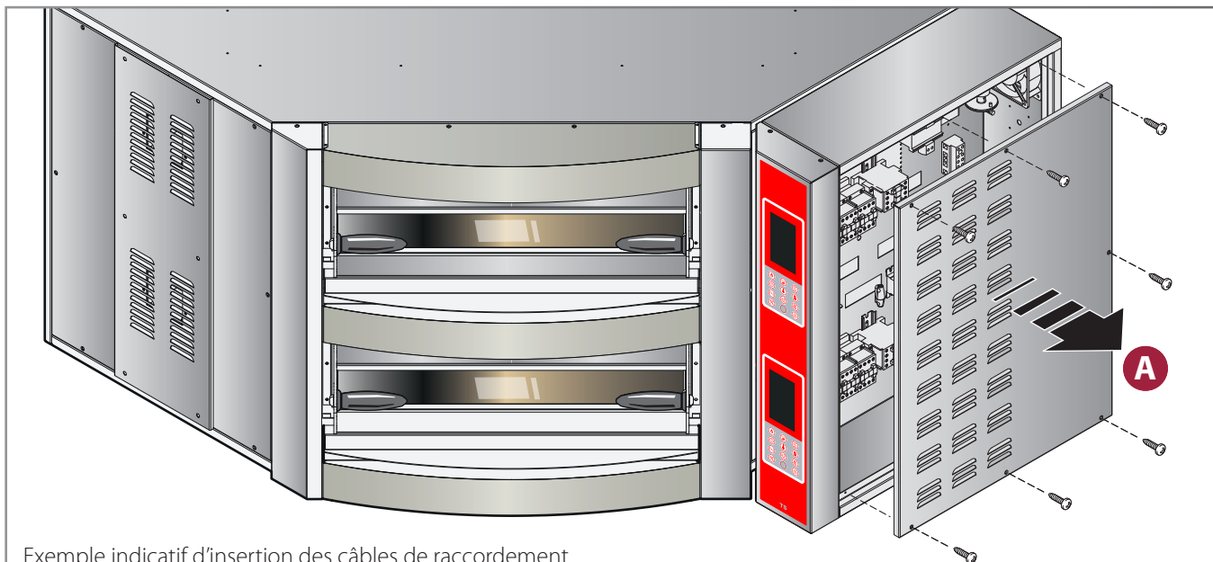
Exemple indicatif d'insertion des câbles de raccordement
