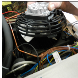
L2. Entfernen Sie den Lüfter, indem Sie ihn gegen den Uhrzeigersinn drehen
