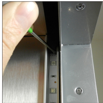
E2. Enlevez les bandes LED defectueuses des rails à l'aide d'un tournevis
