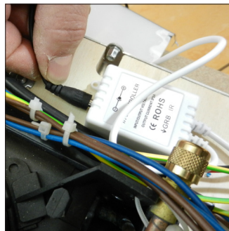
F2. Dèbrancher l'alimentateur, la connection des LED et extraire le récepteur infrarouge par l'ouverture dans la cuve
