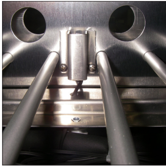
H3. Remettez la sonde et sa la couverture faisant passer le fil par le trou prévu dans la poutre inférieure
