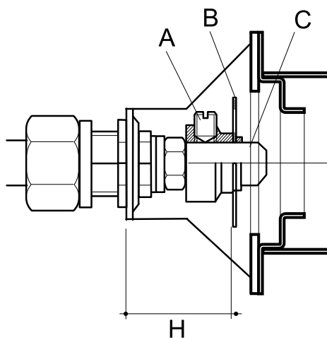
figura A – Inyector del quemador
