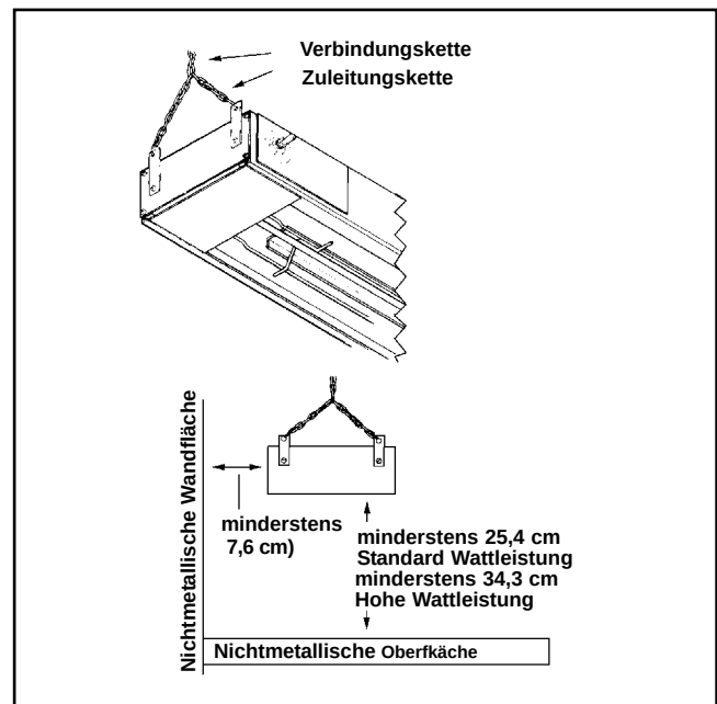
Abbildung 1. Kettenaufhängung
