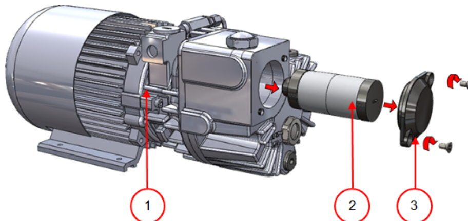
Schéma 22: Remplacement du filtre à échappement d'air
