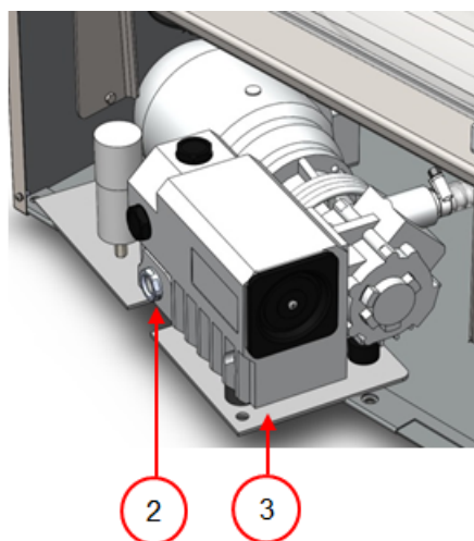
Schéma 21: Plaque de montage TA 52
