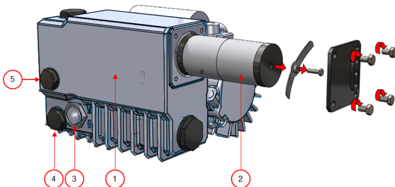
Schéma 20: Aperçu de la pompe
