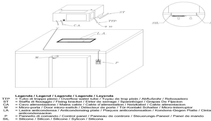
Abbildung 4 – Positionierung der Maschine auf der Zelle.
