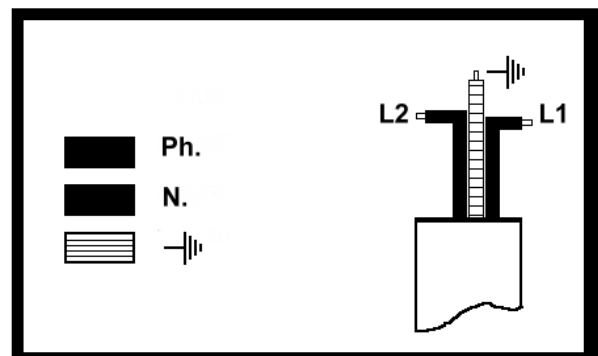
FIG.2 EINPHASIG ANSCHLUSS
