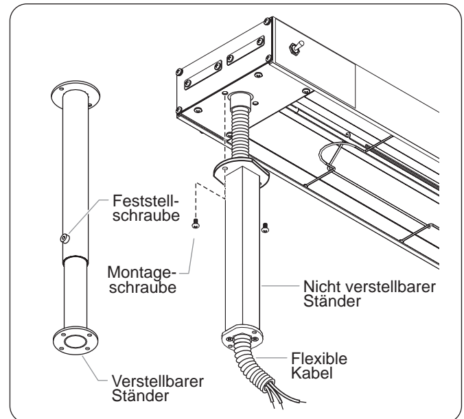
Abbildung 19. Montage auf Ständern
