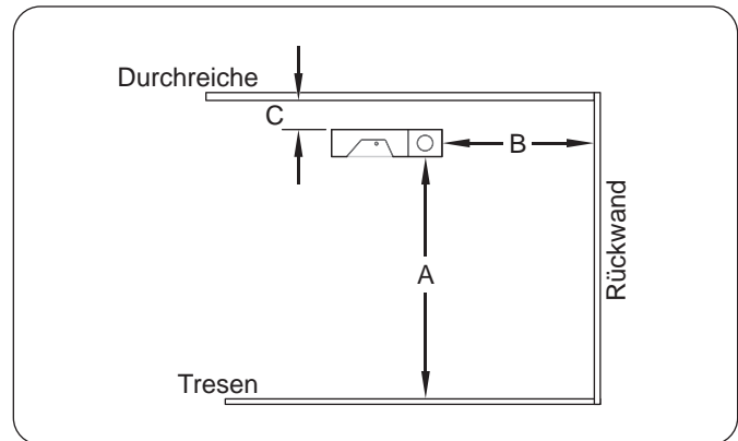
Abbildung 12. Mindestabstände bei nicht entzündbaren Umgebungen
