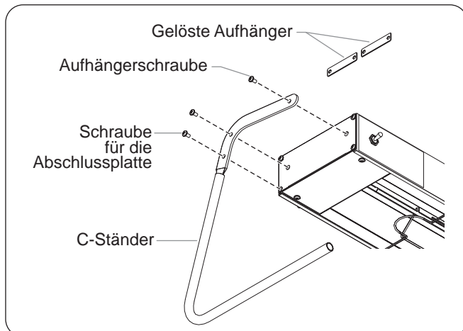
Abbildung 14. C-Ständer
