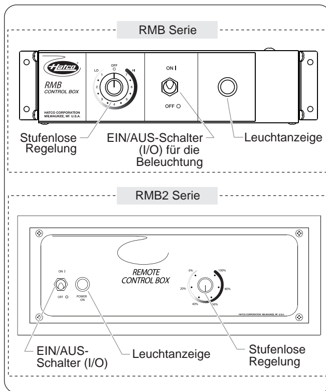
Abbildung 26. Fernbedienungsgehäuse
