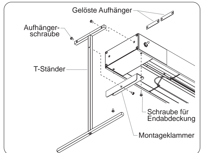
Abbildung 16. Endmontage auf T-Ständern
