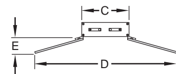
Einzelgeräte (mit optionalen Schutzhauben gezeigt)
