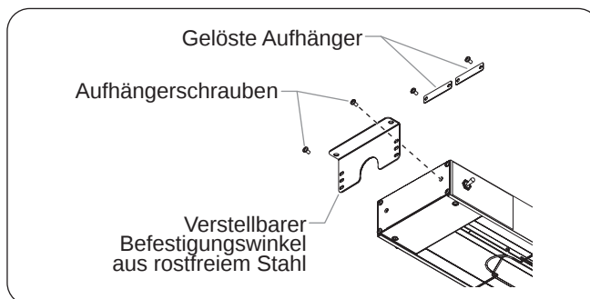
Abbildung 23. Anbringen der verstellbaren Befestigungswinkel an Modellen aus rostfreiem Stahl
