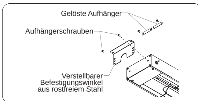
Abbildung 23. Anbringen der verstellbaren Befestigungswinkel an Modellen aus rostfreiem Stahl
