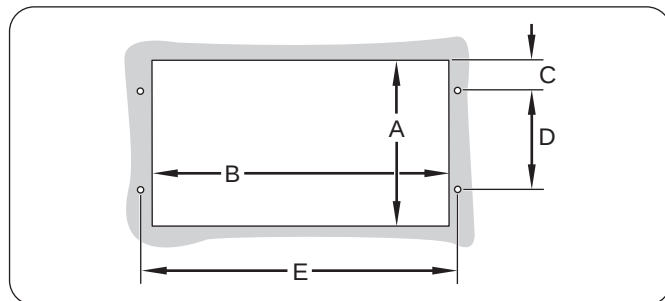
Abbildung 30. Äußere Abmessungen der RMB2-Serie
