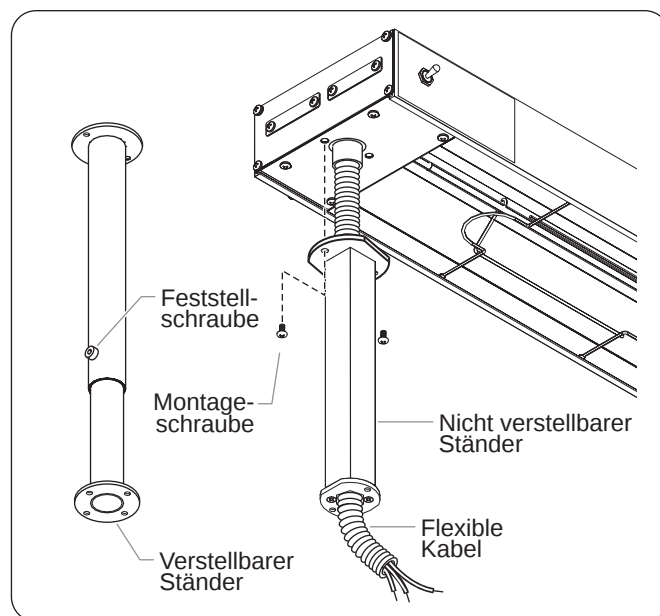
Abbildung 19. Montage auf Ständern
