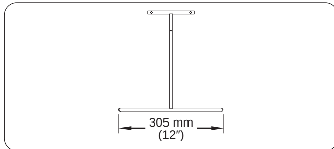
Abbildung 15. Abmessungen der T-Ständer-Füße
