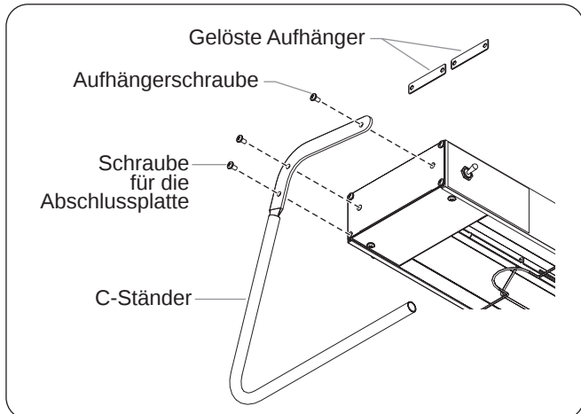
Abbildung 14. C-Ständer
