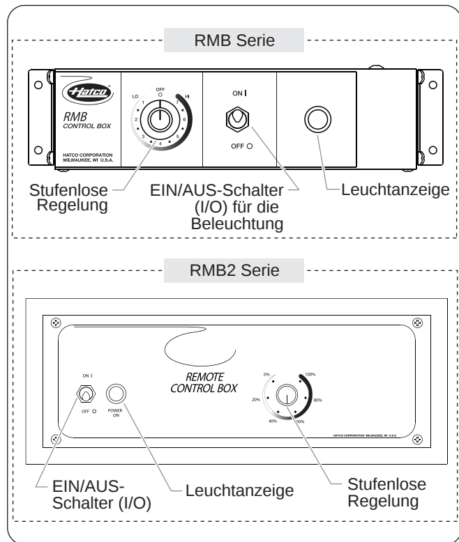
Abbildung 26. Fernbedienungsgehäuse
