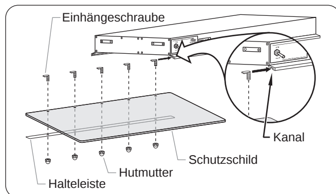
Abbildung 27. Anbau der Schutzhauben
