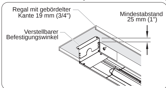
Abbildung 20. Anbringen an einem gebördelten Regal
