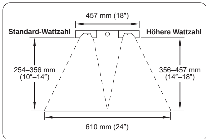
Abbildung 10. Empfohlene Elementhöhe für die Doppelgeräte der Serien GRA-D, GRAH-D, GRAL-D und GRAHL-D mit 152-mm-Abstandhalter (6 Zoll) in allen Längen.
