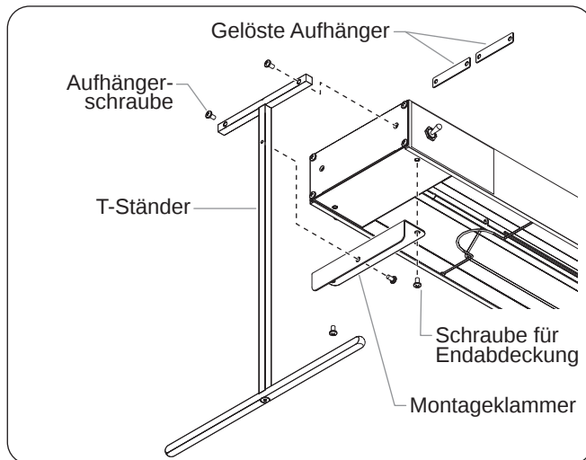
Abbildung 16. Endmontage auf T-Ständern
