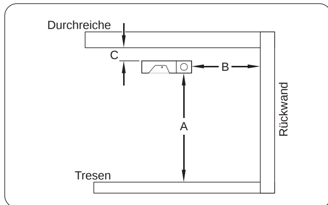
Abbildung 11. Mindestabstände bei entzündbaren Umgebungen
