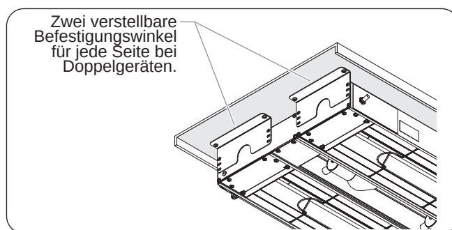
Abbildung 22. Anbringen von Doppelgeräten
