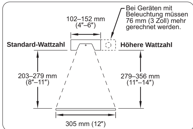
Abbildung 8. Empfohlene Elementhöhe für die Modelle der Serien GR, GRA, GRH, GRN, GRAH, GRAL, GRNH und GRAHL aller Längen (mit Ausnahme von Doppelgeräten).
