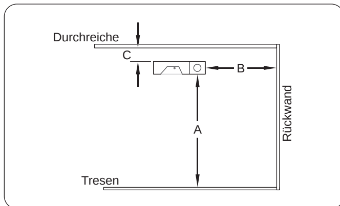
Abbildung 12. Mindestabstände bei nicht entzündbaren Umgebungen
