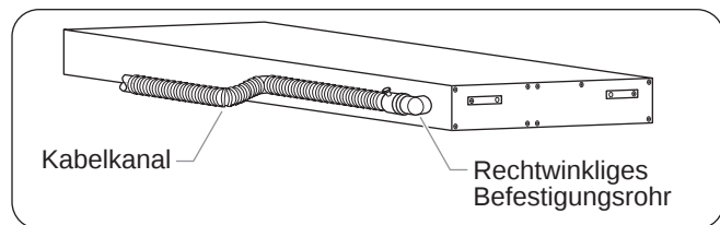
Abbildung 24. Anschluss des Kabelkanals
