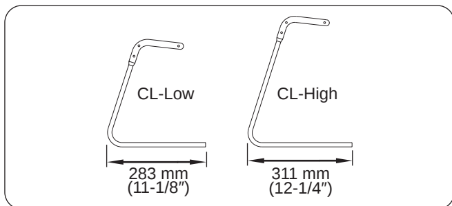
Abbildung 13. Abmessungen der C-Ständer-Füße
