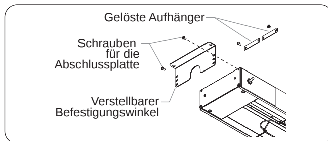
Abbildung 21. Anbringen der verstellbaren Befestigungswinkel
