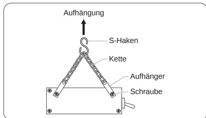
Abbildung 17. Montage mit S-Haken
