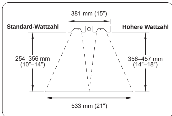
Abbildung 9. Empfohlene Elementhöhe für die Doppelgeräte der Serien GRA-D, GRAH-D, GRAL-D und GRAHL-D mit 76-mm-Abstandhalter (3 Zoll) in allen Längen.
