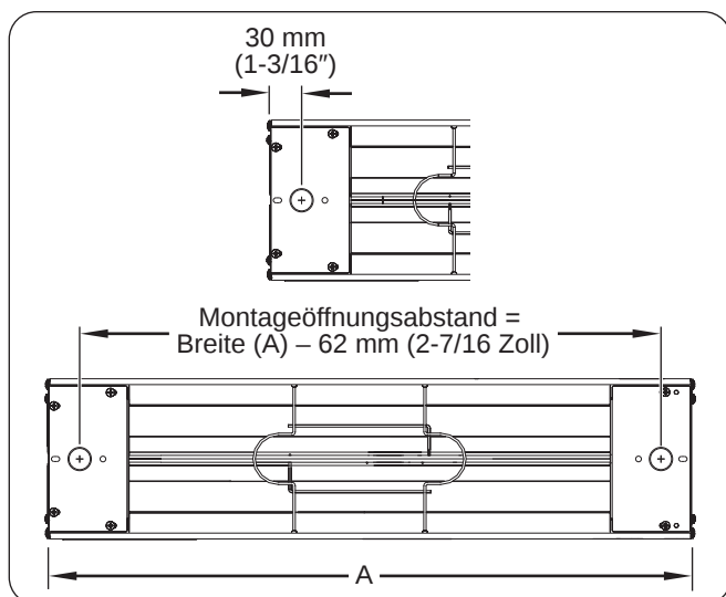
Abbildung 18. Abmessungen für Kabelkanal in Arbeitsplatte
