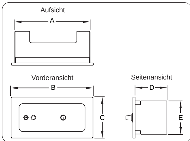
Abbildung 29. Abmessungen der RMB2-Serie
