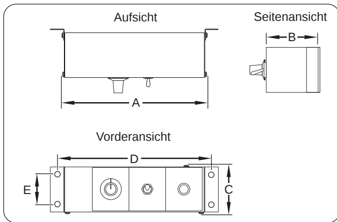
Abbildung 28. Abmessungen der RMB-Serie
