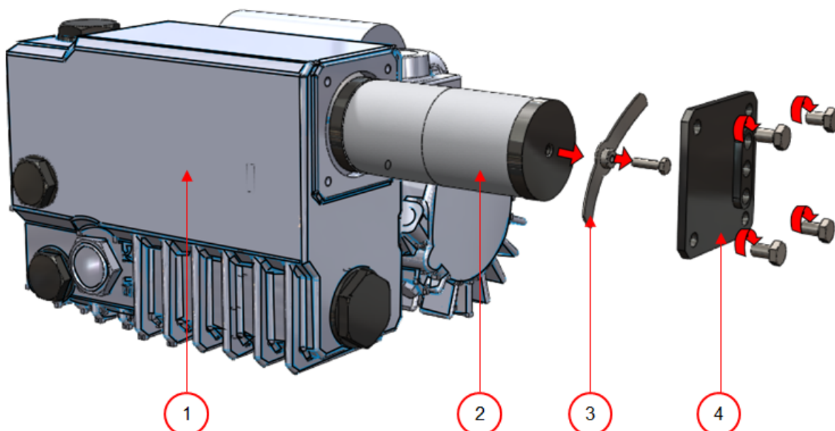
Abbildung 18: Austausch des Ölnebelfilters (Pumpe 16/21 m 3 )
