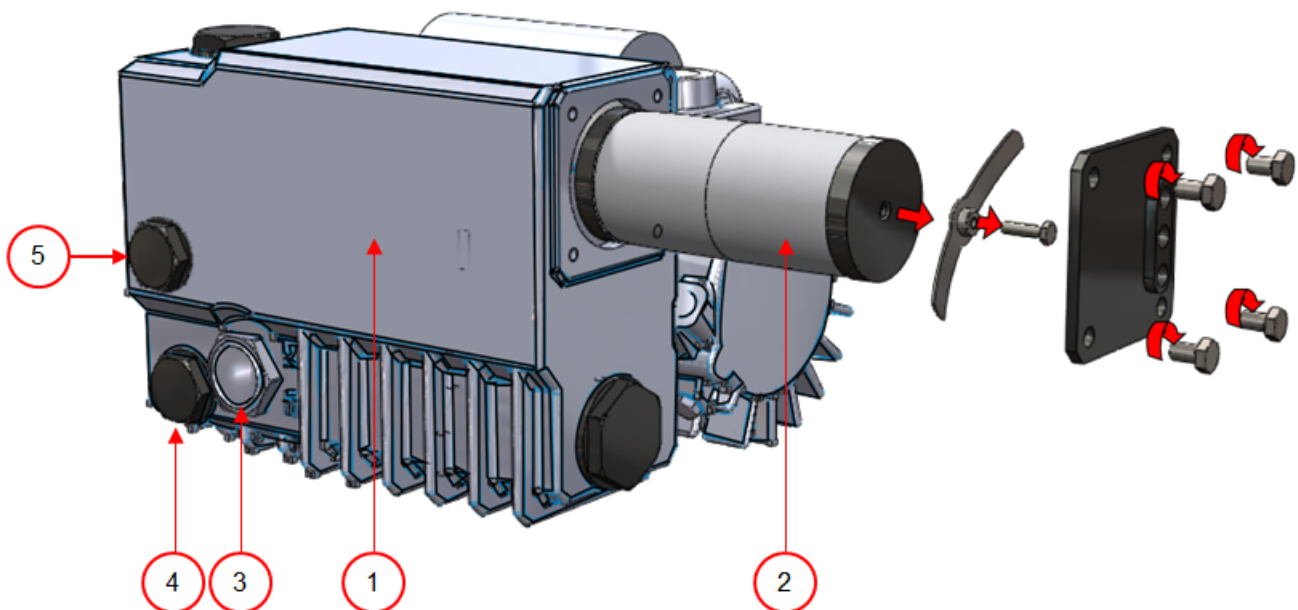
Abbildung 4: Übersicht über die Pumpe (Pumpe 16 m 3 )
