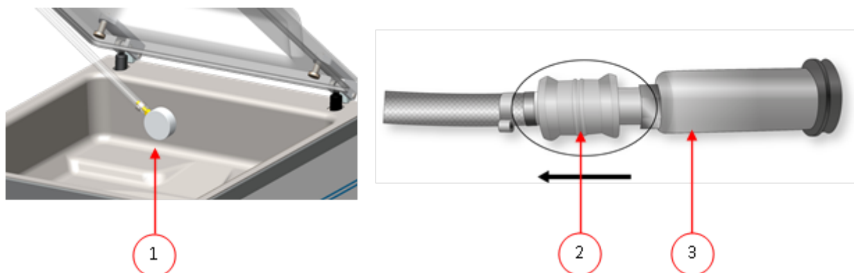
Abbildung 14: Adaptersatz für Externes Vakuumieren (ACS)
