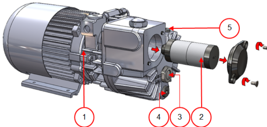
Abbildung 3: Übersicht über die Pumpe (Pumpe 8 m 3 )
