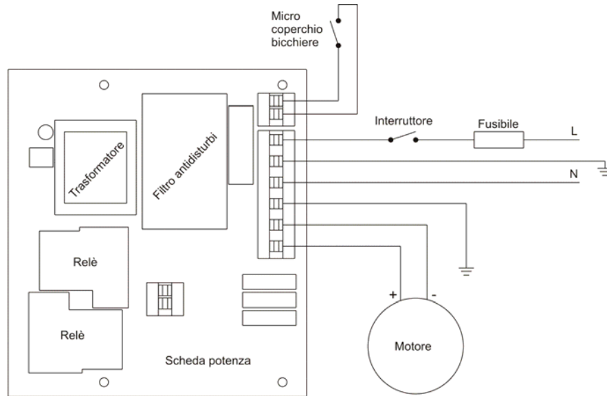
Abb. 5 - Elektroplan
