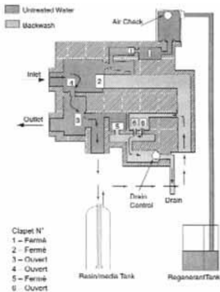
Position C1 - Détassage I
