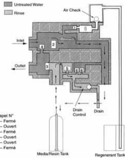
Position C5 - Rinçage rapide I
