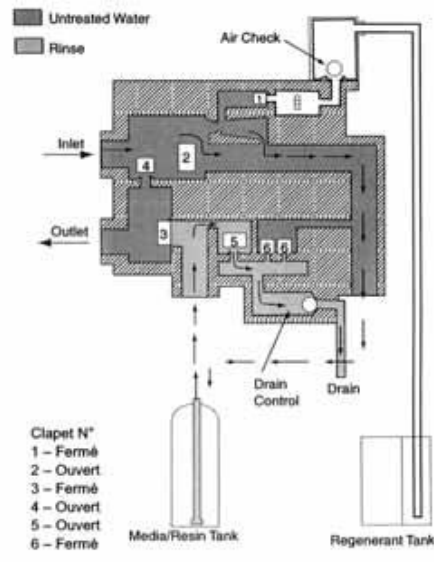
Position C8 - Remplissage
