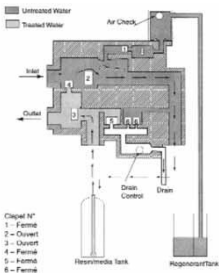
Position Eau traitée C0 (fonctionnement normal)
