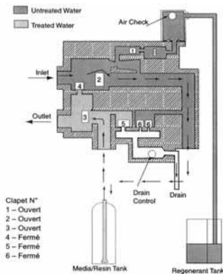
Position C8 - Remplissage
