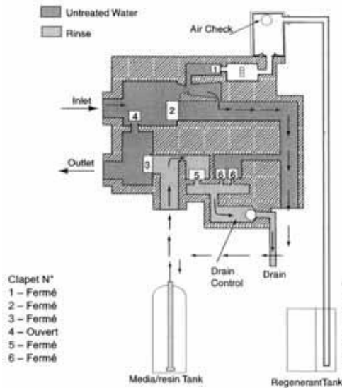
Position C4 - Pause du système (repressurisation)
