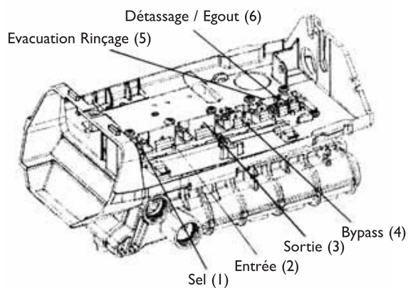
Position Eau traitée C0 (fonctionnement normal)
