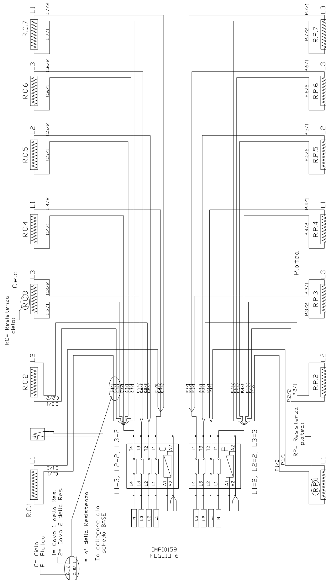
Fig. 9-6 Schéma électrique à 400V 3-N seulement pour modèle Teorema Polis Pw 8 (connexion de puissance)
