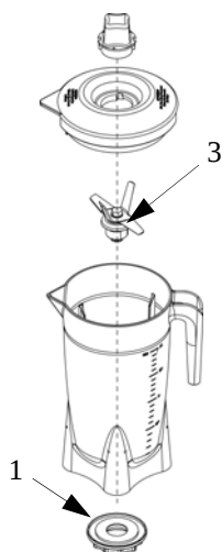
FIG.n°9 - Extraction du porte-couteau
