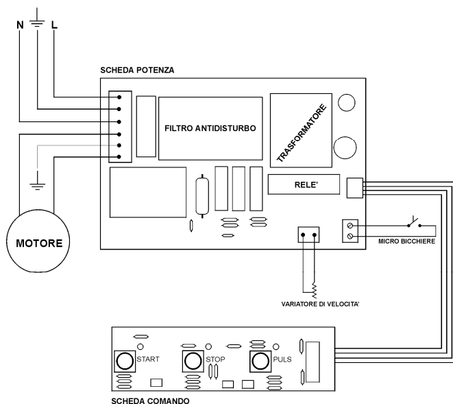
FIG. n°5 - Schéma électrique
