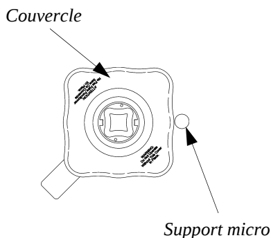
FIG.n°7 - Position du couvercle
