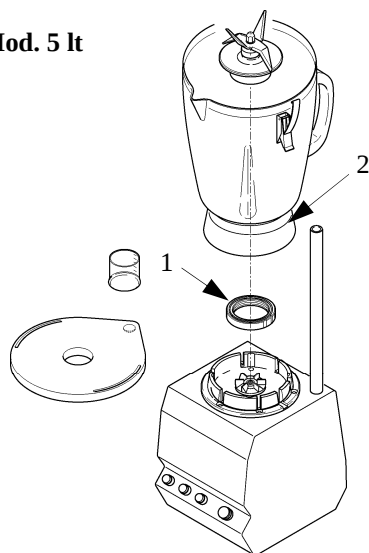
FIG.n°9 - Extraction du porte-couteau
