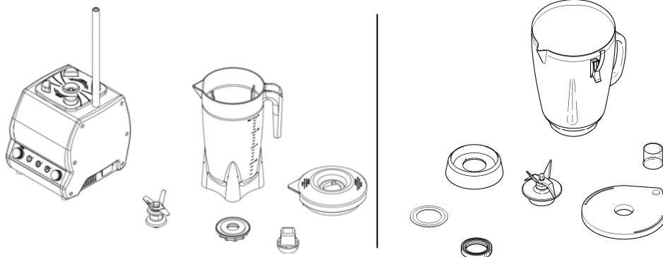
FIG n°10 - Machine démontée pour le nettoyage
