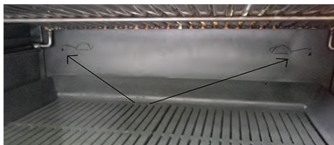
Points de graissage intérieurs du système de levage
