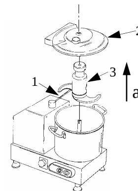
FIG. n°10 - Démontage porte-couteaux
