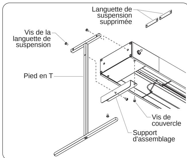
Figure 16. Montage du pied en T à l'extrémité de la rampe
