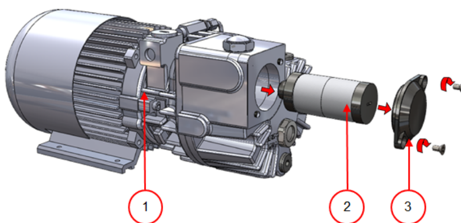
Schéma 17: Remplacement du filtre à échappement d'air (Pompe 8 m 3 )
