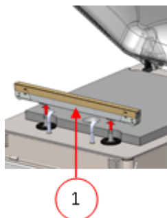
Schéma 19: Retrait de la barre de soudure
