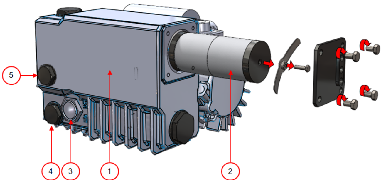
Schéma 4: Aperçu de la pompe (Pompe 16 m 3 )
