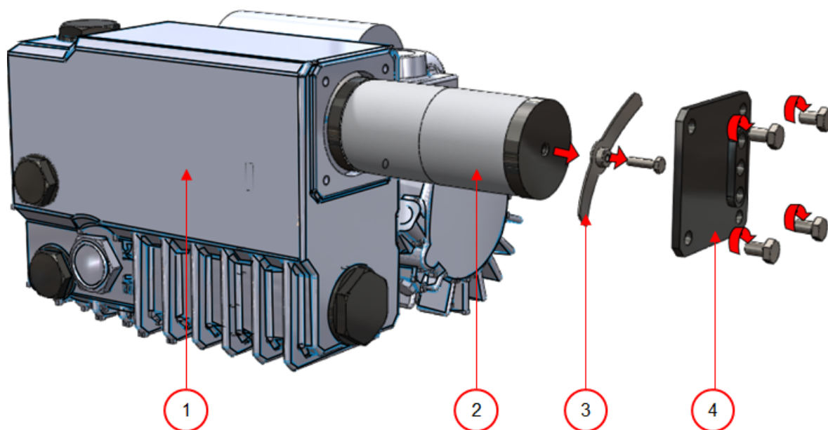
Schéma 18: Remplacement du filtre à échappement d'air (Pompe 16/21 m 3 )
