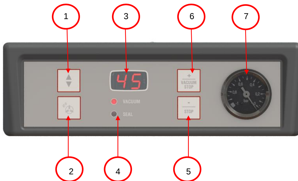
Schéma 7: Panneau de commande du système de commande 1 programme
