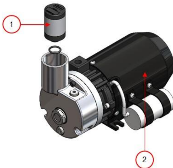
Schéma 10: Remplacement du filtre à échappement d'air (Pompe 4 m 3 /h)
