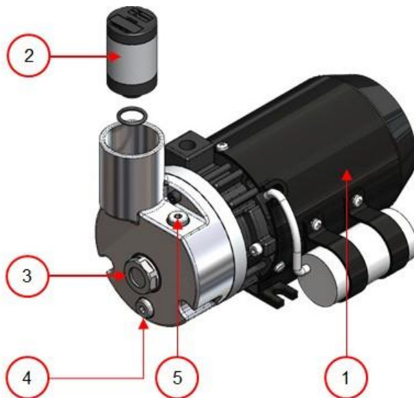
Schéma 3: Aperçu de la pompe (Pompe 4 m 3 /h)
