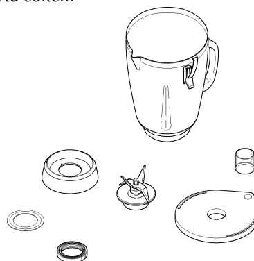
FIG n°10 - Macchina smontata per la pulizia
