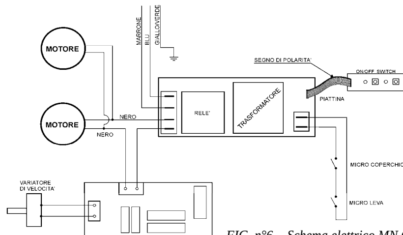
FIG. n°6 - Schema elettrico MN C9VV
