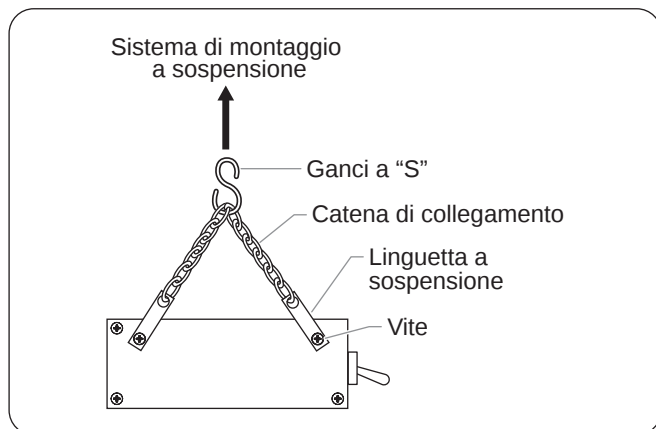
Figura 17. Montaggio con ganci a "S"
