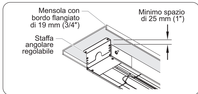
Figura 20. Installazione su una mensola con bordi flangiati
