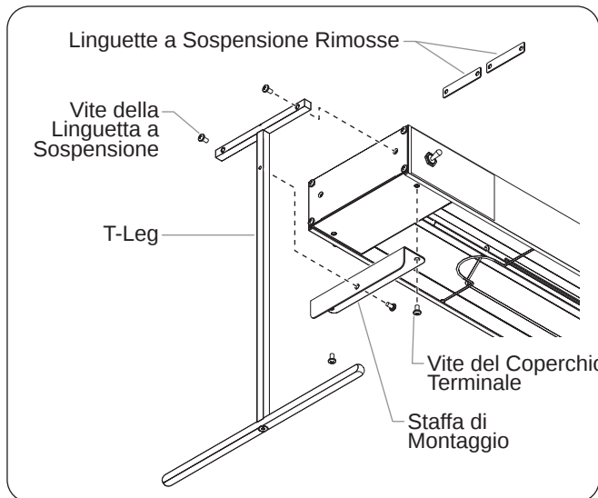
Figura 16. Montaggio terminale del supporto T-Leg
