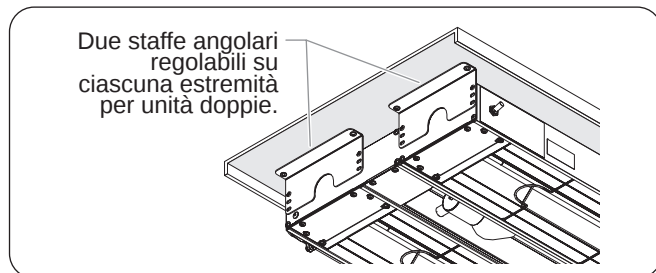
Figura 22. Montaggio unità doppia
