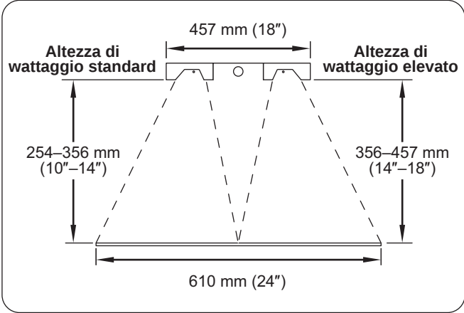
Figura 10. Altezza degli elementi consigliata per i modelli doppi GRA-D, GRAH-D, GRAL-D e GRAHL-D con un distanziale di 152 mm (6") in tutte le lunghezze.
