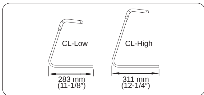
Figura 13. Dimensioni dell'ingombro del C-Leg
