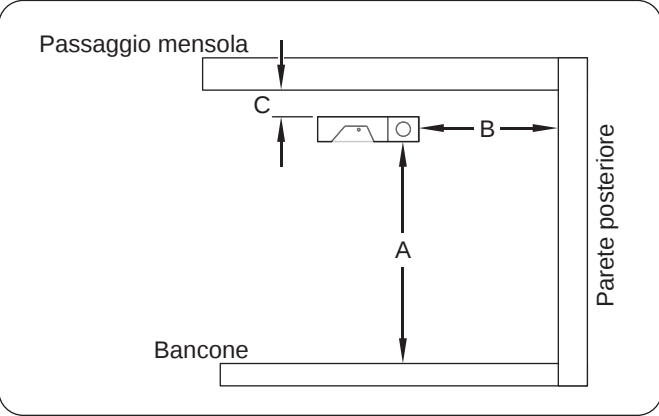
Figura 11. Requisiti di distanza per combustibili NOTA: Le dimensioni dei modelli di riscaldamento variano in base all'altezza dell'unità.
