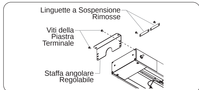
Figura 21. Installazione della staffa angolare regolabile su modello in alluminio
