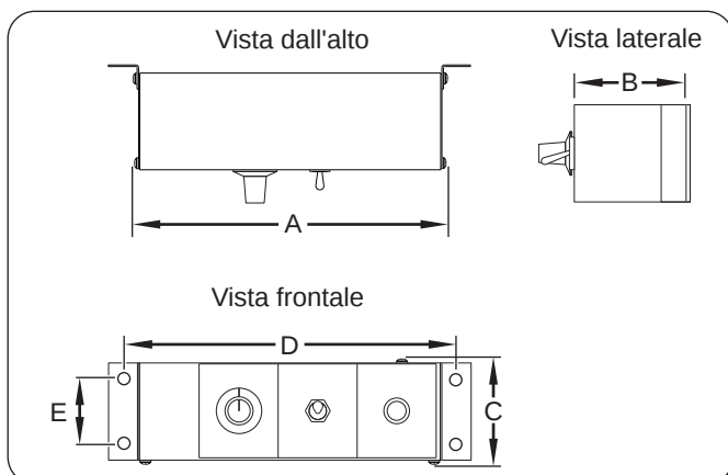
Figura 28. Dimensioni Serie RMB
