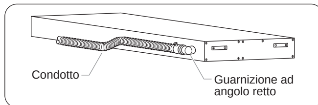
Figura 24. Collegamenti del condotto
