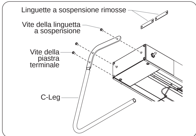
Figura 14. Supporto C-Leg
