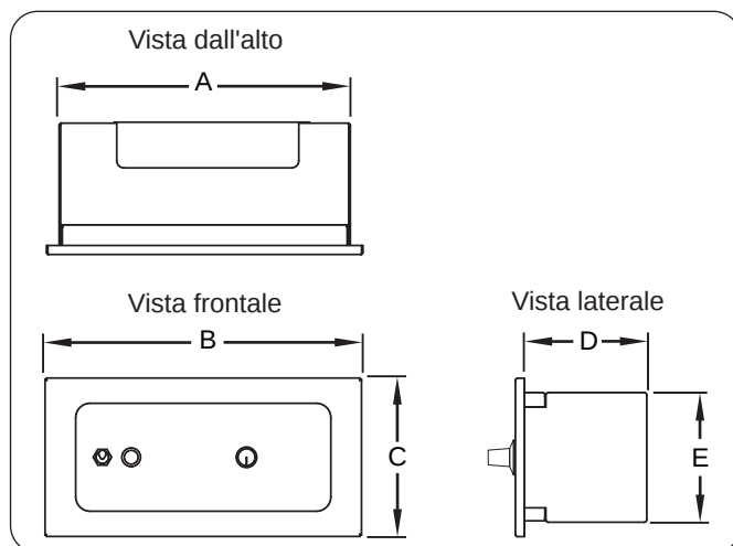
Figura 29. Dimensioni Serie RMB2
