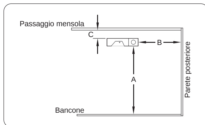
Figura 12. Requisiti di distanza per non combustibili
