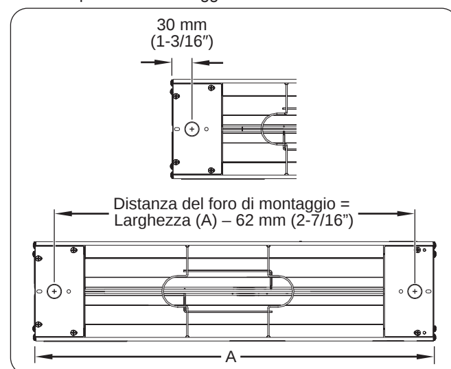
Figura 18. Dimensione del foro del condotto del piano di lavoro
