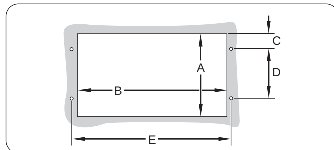
Figura 30. Dimensioni interruttori Serie RMB2
