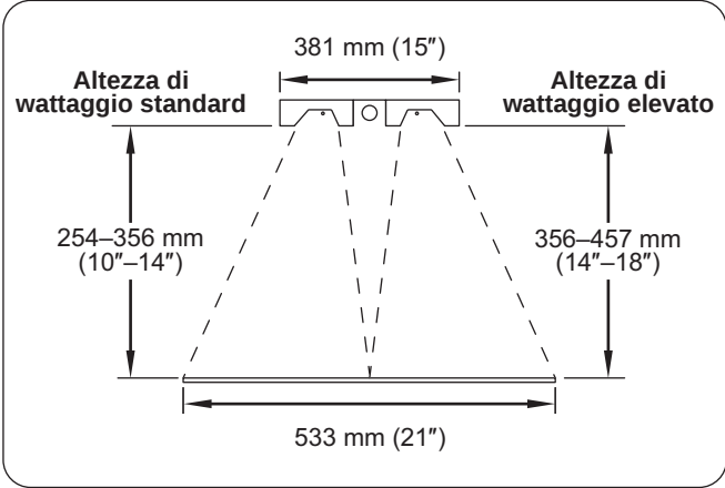
Figura 9. Altezza degli elementi consigliata per i modelli doppi GRA-D, GRAH-D, GRAL-D e GRAHL-D con un distanziale di 76 mm (3") in tutte le lunghezze.
