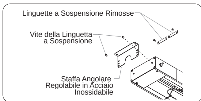
Figura 23. Installazione della staffa angolare regolabile su modello in acciaio inossidabile
