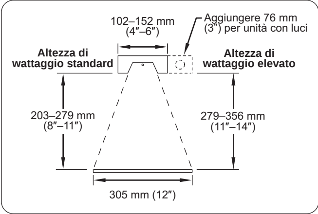
Figura 8. Altezza degli elementi consigliata per i modelli GR, GRA, GRH, GRN, GRAH, GRAL, GRNH e GRAHL in tutte le altezze (modelli doppi esclusi).
