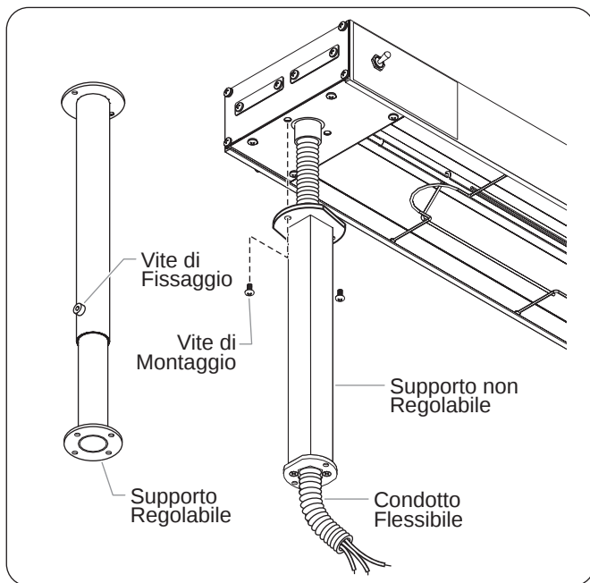
Figura 19. Montaggio su supporto tubolare
