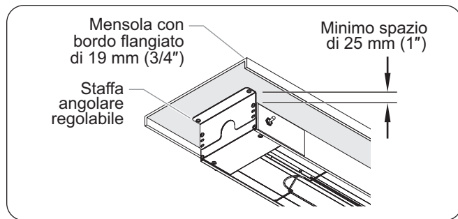
Figura 20. Installazione su una mensola con bordi flangiati
