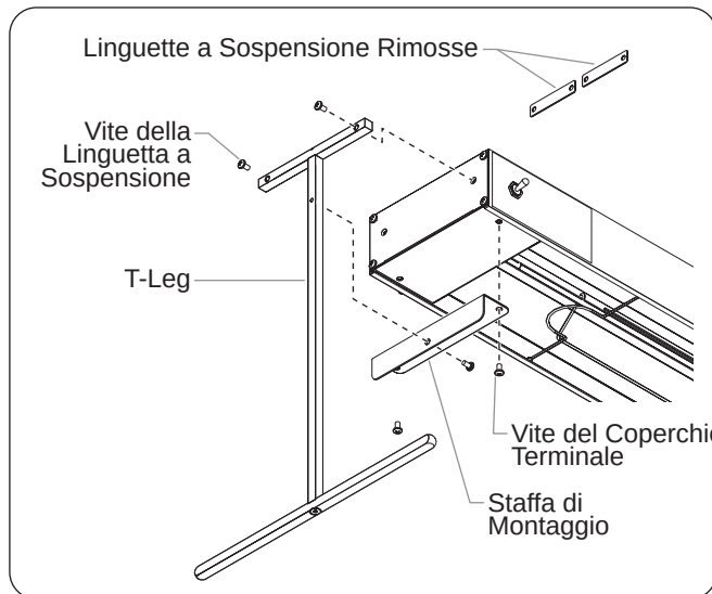
Figura 16. Montaggio terminale del supporto T-Leg
