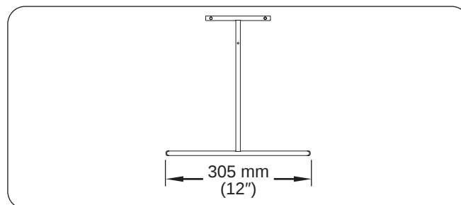
Illustratie 15. Afmetingen oppervlak T-vormig onderstel
