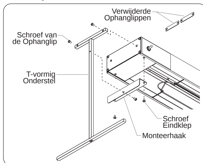
Illustratie 16. Eindmontage met T-vormig onderstel
