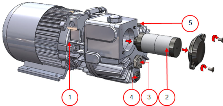
Figuur 3: Overzicht van de pomp (pomp 8 m 3 )
