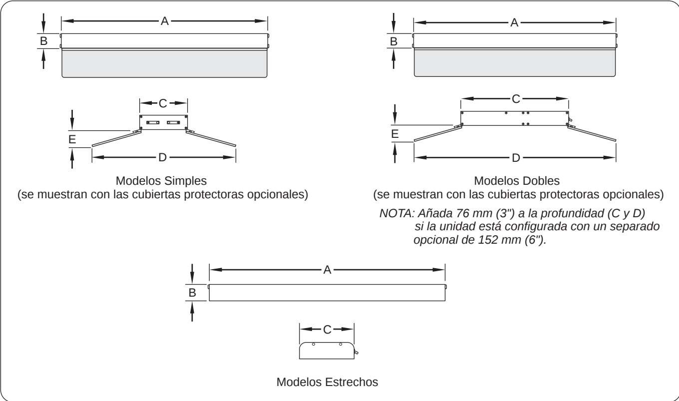
Figura 7. Dimensiones
