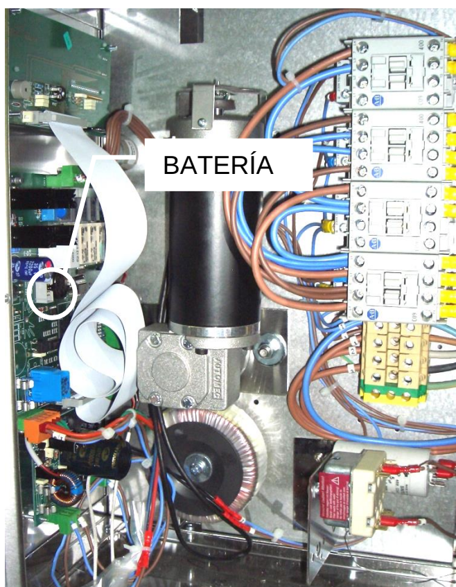
Fig. 8.1 Cuadro comandos, posición BATERÍA.
