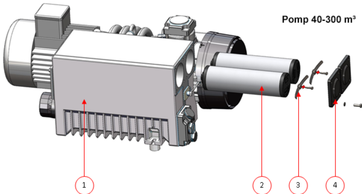
Figura 17: Sustitución del filtro de salida de aceite (bomba de 40-300 m 3 )
