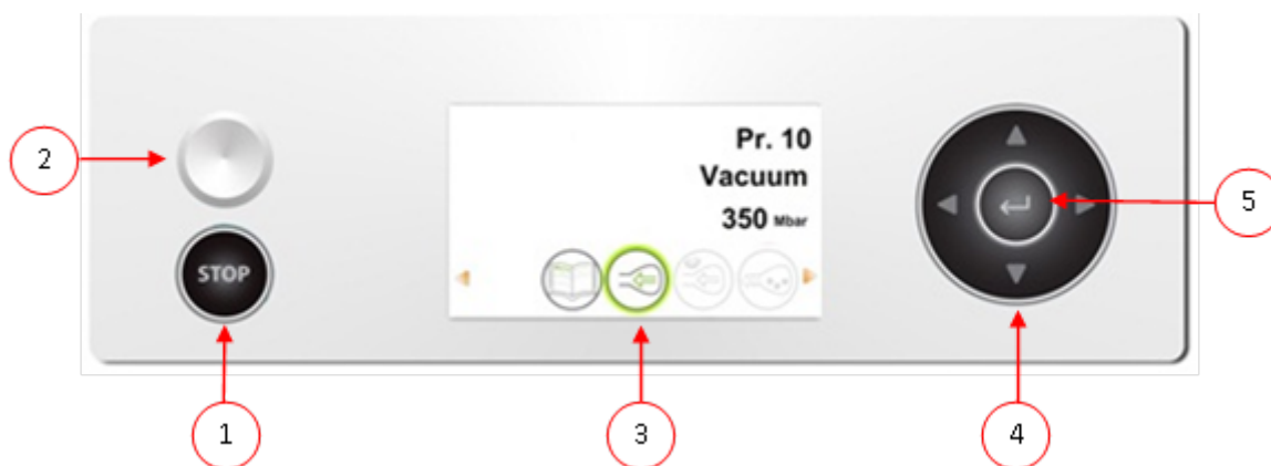
Figura 7: Panel de control del sistema de control de avanzado (ACS)
