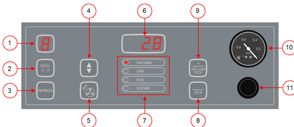
Figura 6: Panel de control del sistema de control de 10 programas
