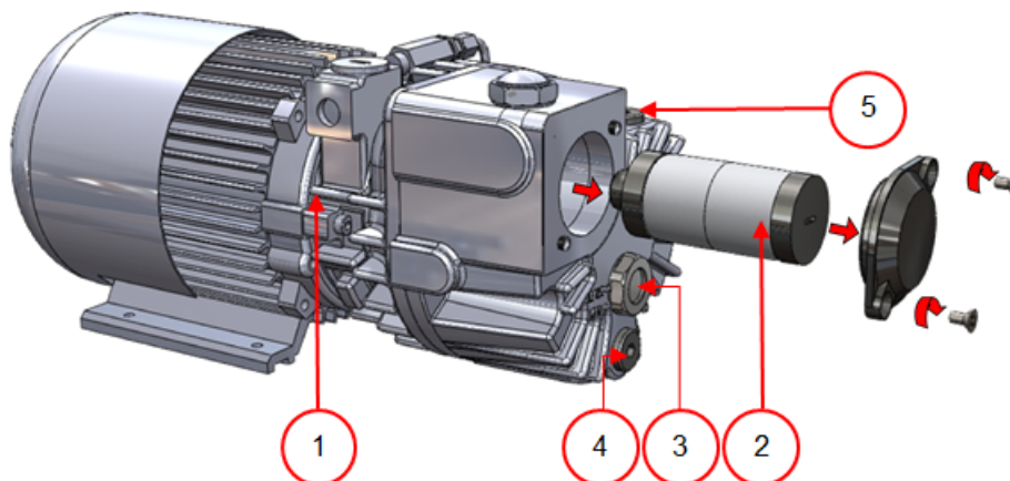
Figura 3: Descripción general de la bomba (bomba 8 m 3 )
