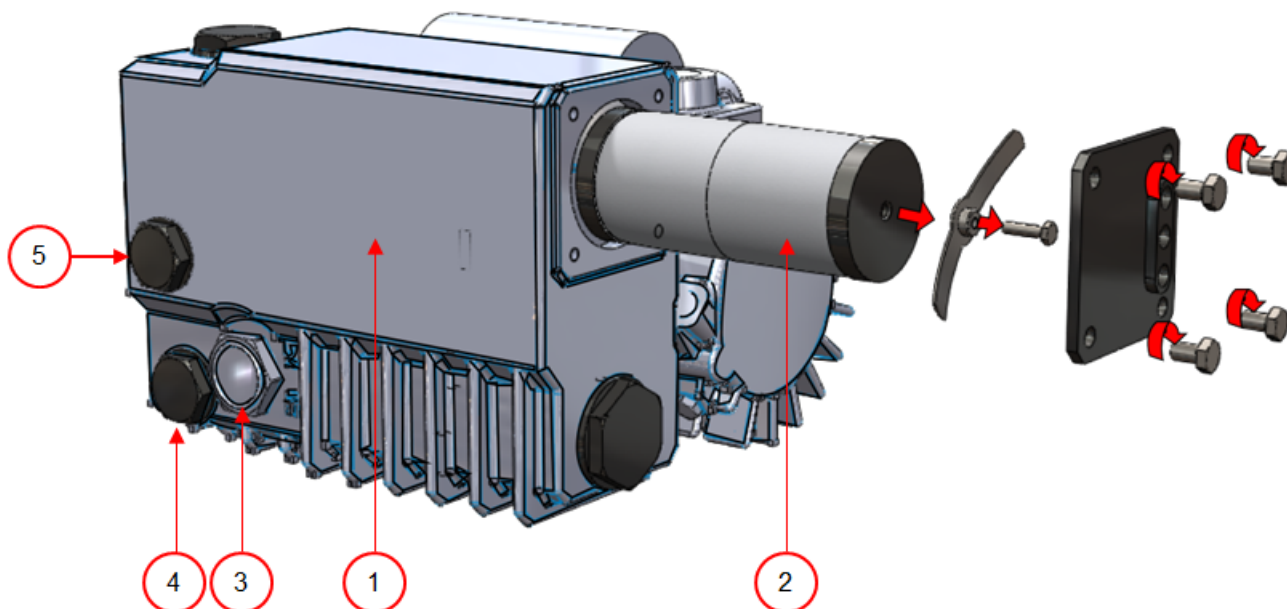
Figura 4: Descripción general de la bomba (bomba 16 m 3 )
