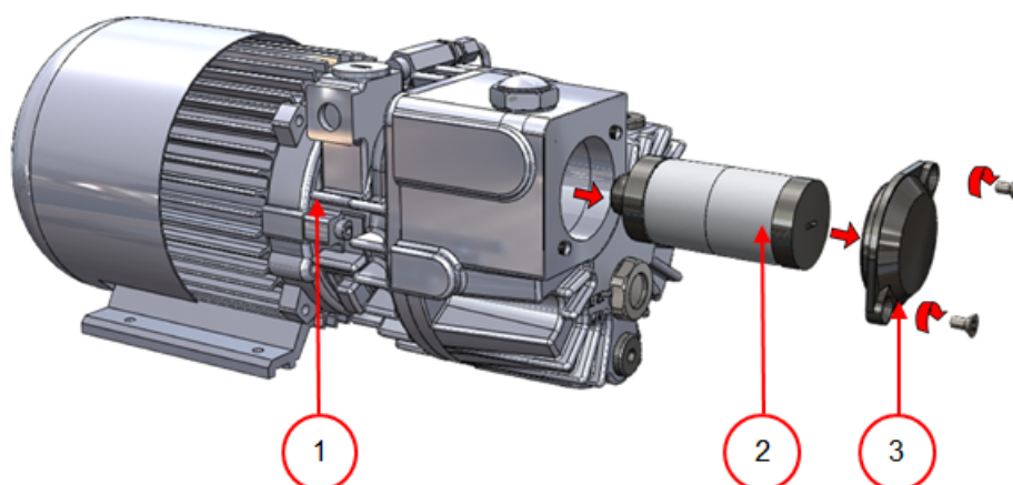
Figura 17: Sustitución del filtro de salida de aceite (bomba de 8 m 3 )
