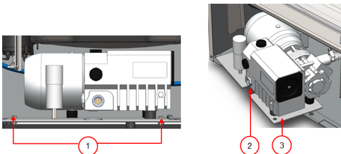
Figura 16: Placa de montaje del modelo Boxer 52
