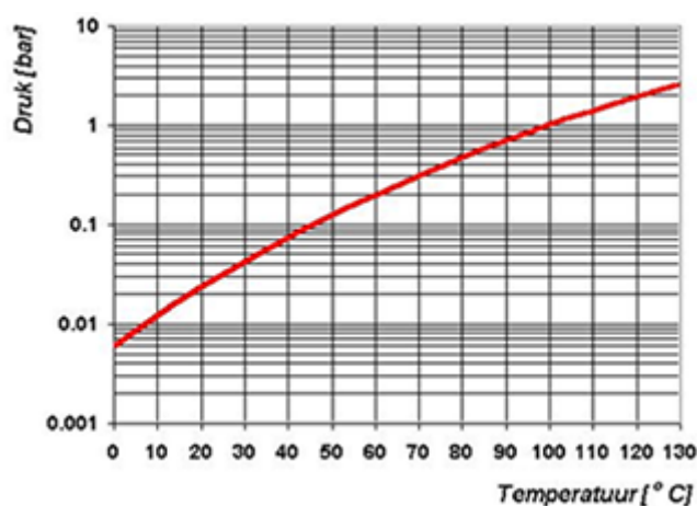
Figura 15: Curva de presión de vapor del agua
