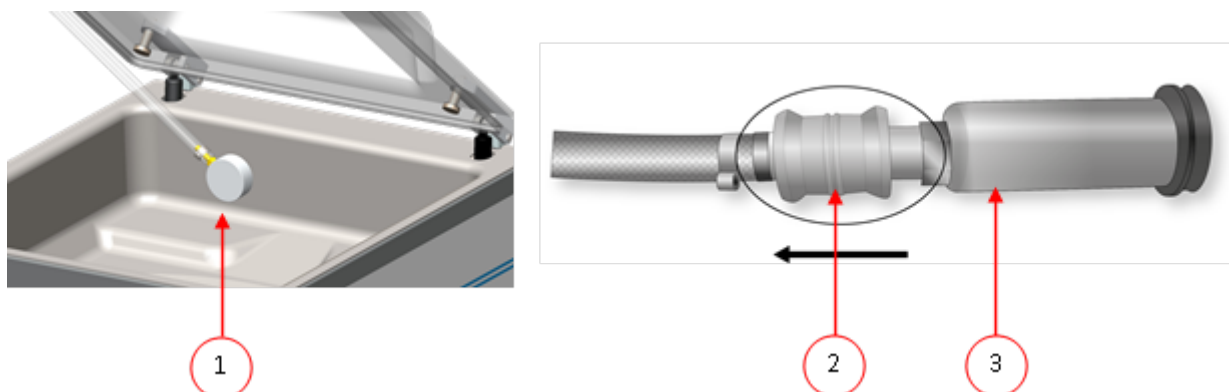
Figura 12: Juego de adaptador de vacío externo (sistema de control de 10 programas)
