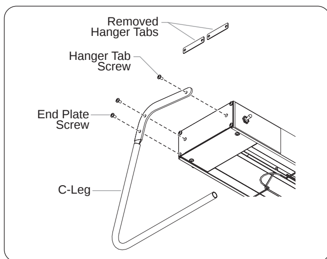
Figure 14. C-Leg Stand
