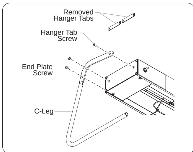
Figure 14. C-Leg Stand
