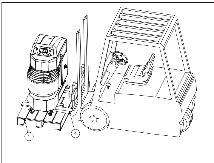
Fig. 2 Transport de la machine.
