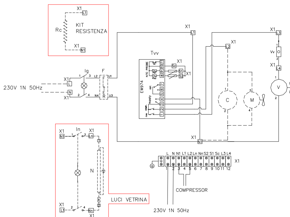
Fig. 2: SCHEMA ELETTRICO ñ WIRING DIAGRAM ñ SCHALTPLAN - SCHEMA ELECTRIQUE ELEMENTI REFRIGERATI PREDISPOSTI PER GRUPPO REMOTO
